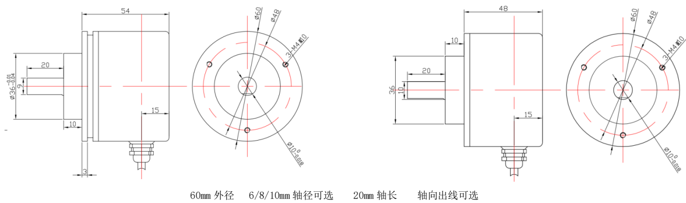
夹紧同步法兰 （ 电缆输出或插头输出可选 ）
