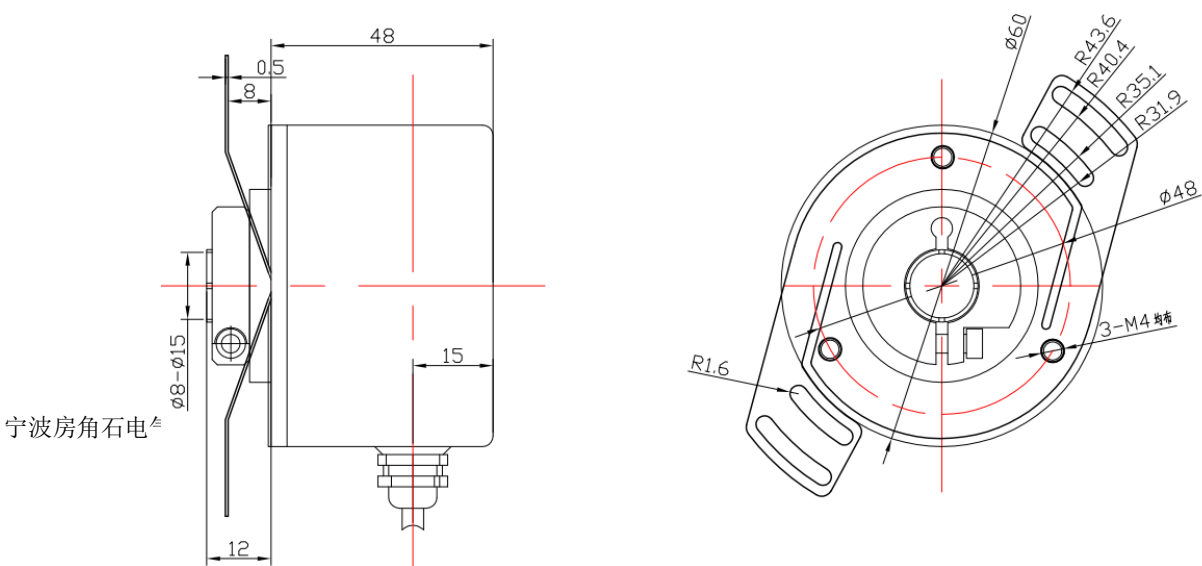
盲孔型/半通孔法兰 （ 电缆输出或插头输出可选 ）
